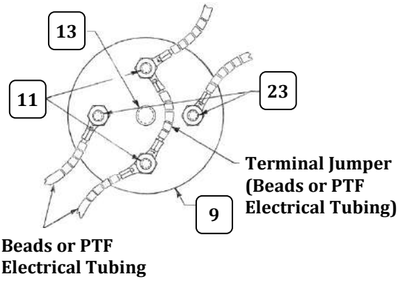
Terminal Wiring
